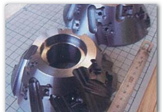
鋼材の開先加工用カッター受注製作
