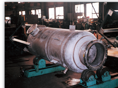
ステンレス製圧力容器 φ1200×2500L
