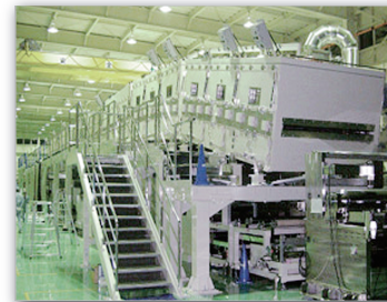
Film装置
