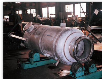
ステンレス製圧力容器 φ1200×2500L
