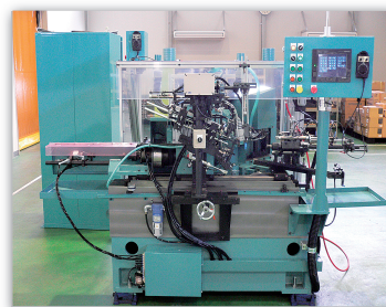
研削機
