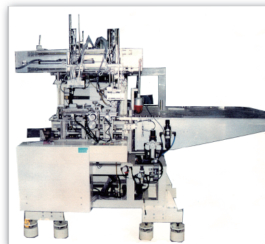
液晶セルピン挿入機
